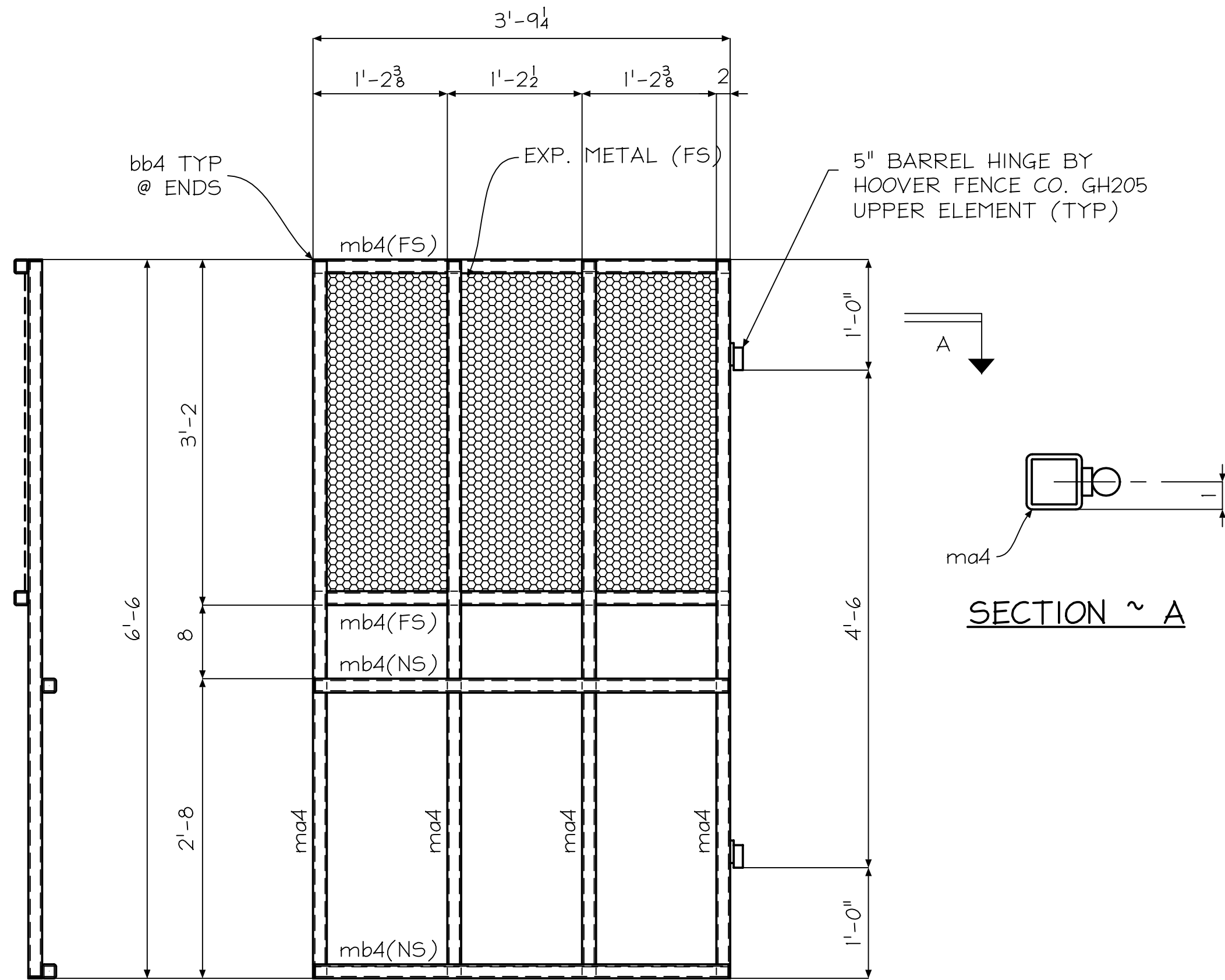
1 - FRAME - 4MI
