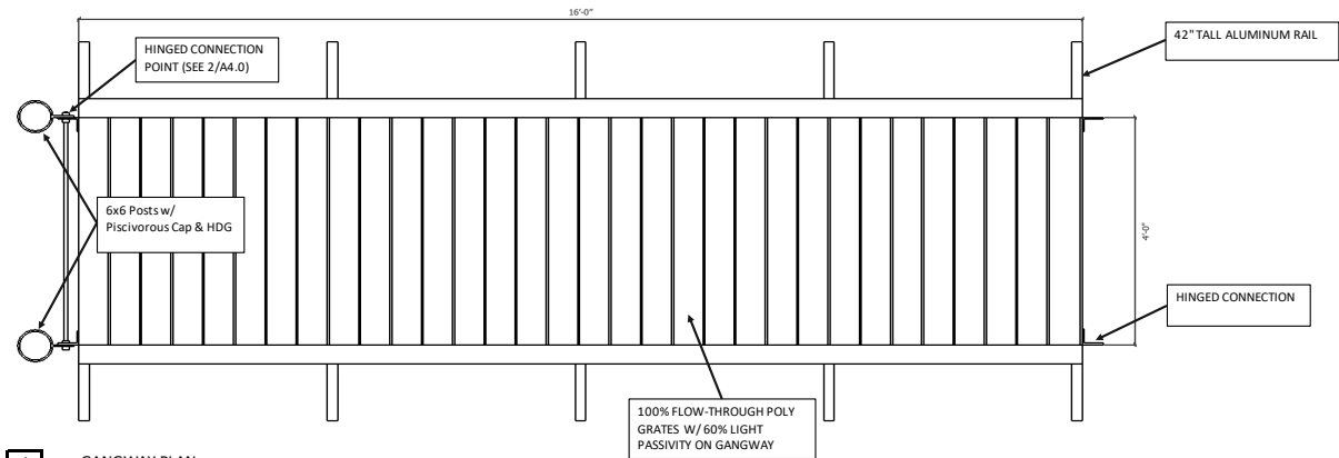
1 GANGWAY PLAN NTS
