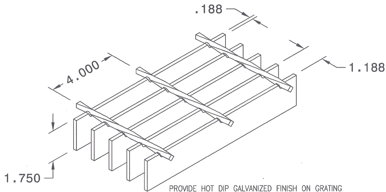
04 TRENCH DRAIN GRATING DETAIL N.T.S.
