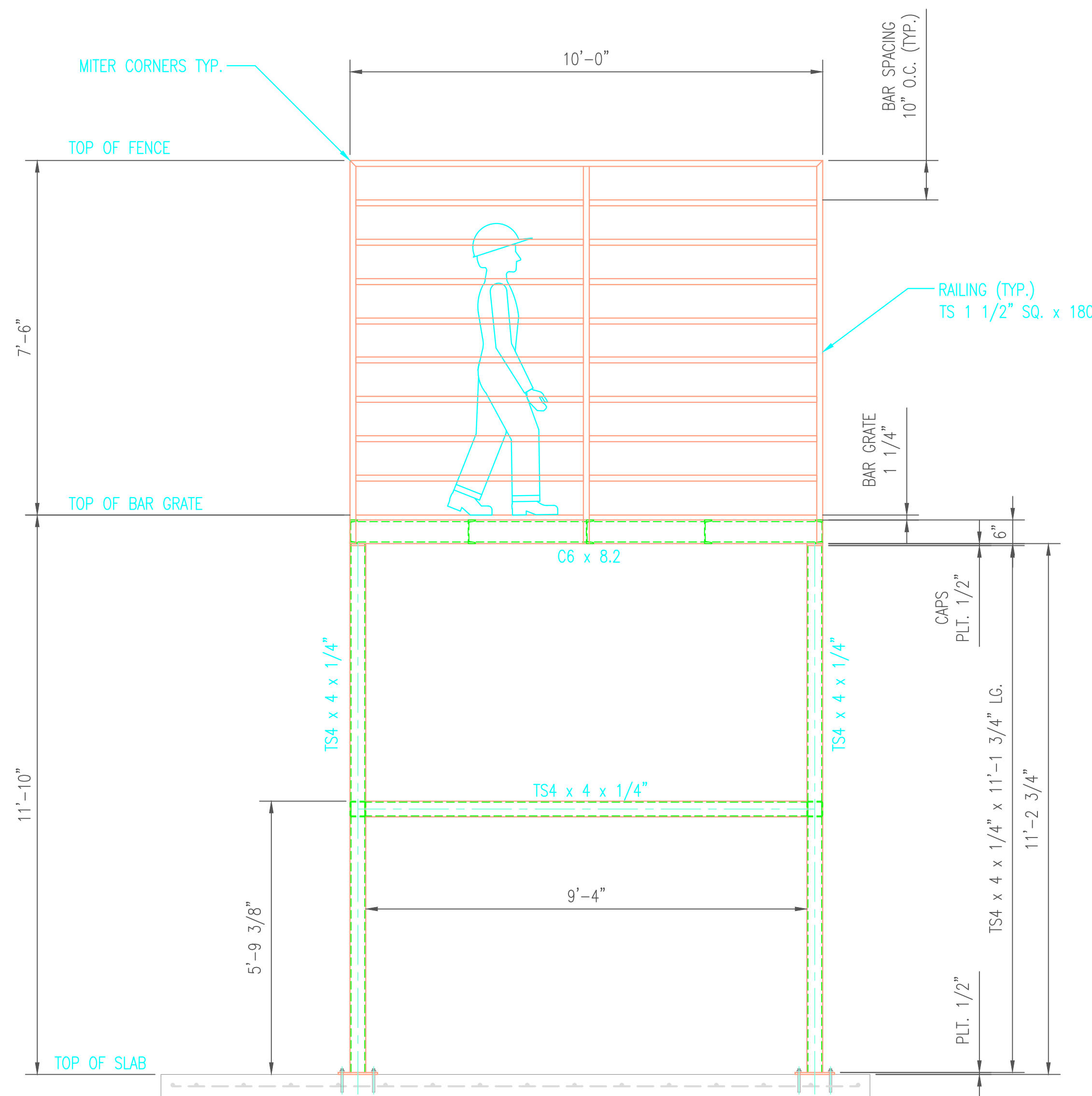
ELEVATION
