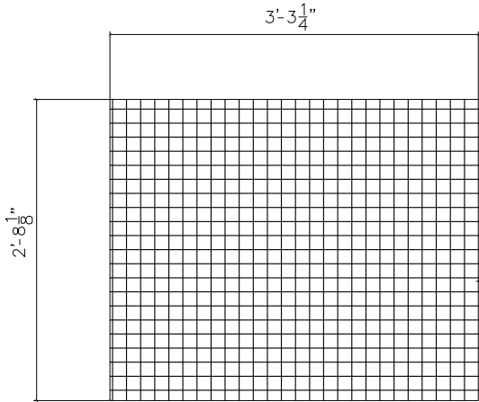
GR1-8GA 1 1/2"SQ. WOVEN WIRE MESH 2-REQ
