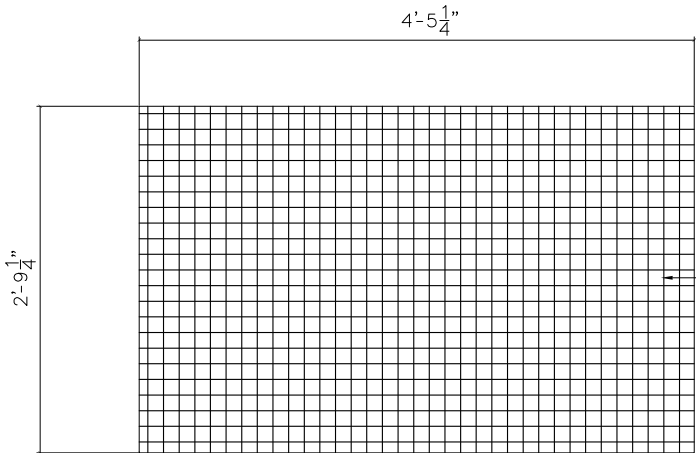
GR2A-8GA 1 1/2"SQ. WOVEN WIRE MESH 3-REQ
