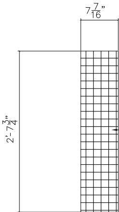
GR4B-8GA 1 1/2"SQ. WOVEN WIRE MESH 1-REQ
