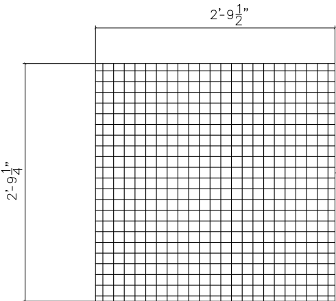
GR3-8GA 1 1/2"SQ. WOVEN WIRE MESH 2-REQ
