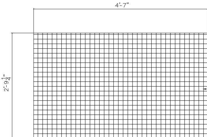
GR2A-8GA 1 1/2"SQ. WOVEN WIRE MESH 2-REQ
