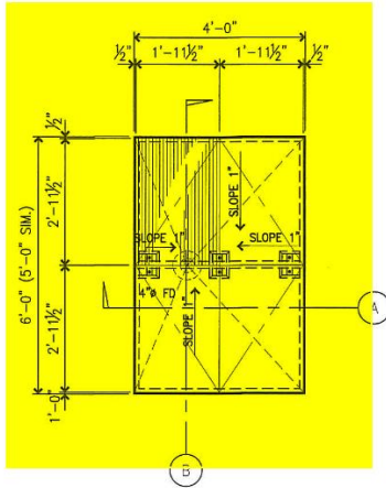
PLAN SCALE: 1/2"=1'-0"
