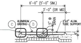
LONGITUDINAL SECTION B SCALE: 3/8"=1'-0"
